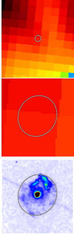
IRAS 60 micron: Infrared (60 micron)
