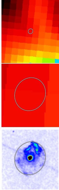
IRAS 100 micron: Infrared (100 micron)
