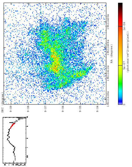
: 4250-6300 eV
